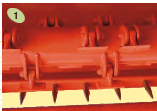
1. Rotore sul quale a scelta si possono montare: mazzette, palette o coltelli 1. Rotor on which can be installed on choice: hammer, blades or knives
