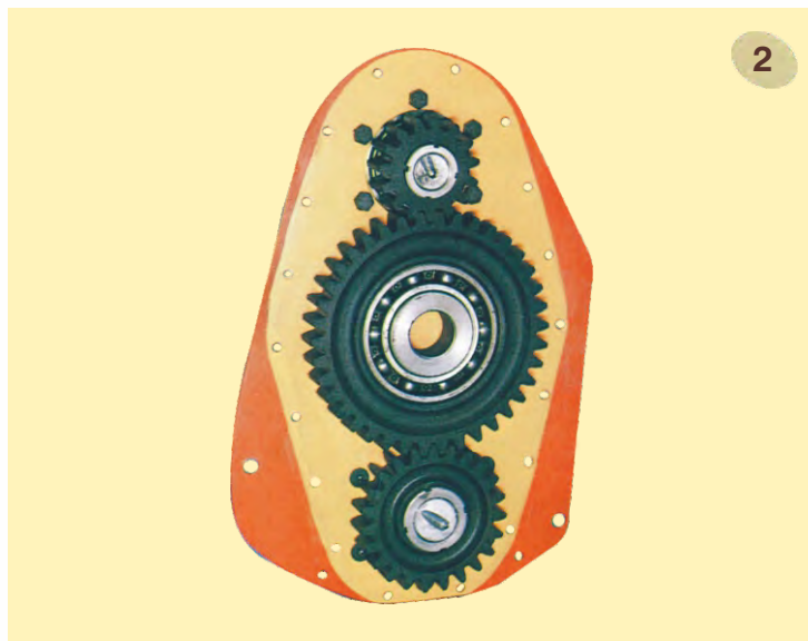
1. Фреза, модель SEL, в версии с гидравлическим смещением 2. Боковая зубчатая трансмиссия
