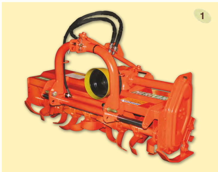
1. Fraiseuse modèle SEL en version avec déplacement hydraulique 2. Transmission latérale à engrenages
